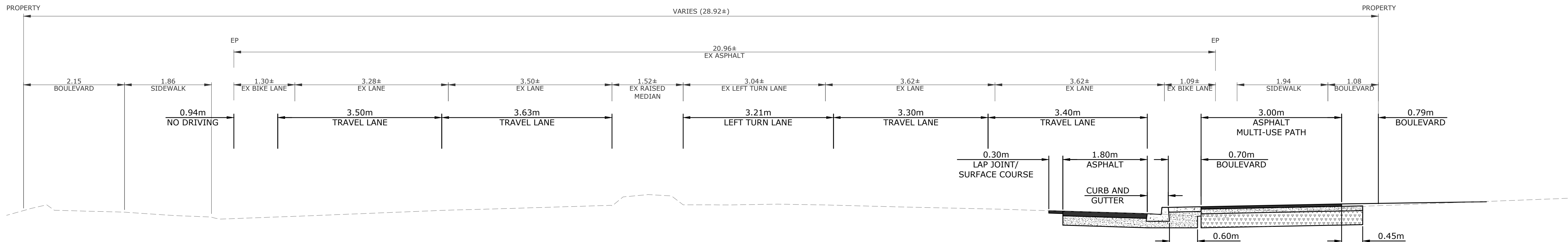
SECTION B-B SCALE: N.T.S.
